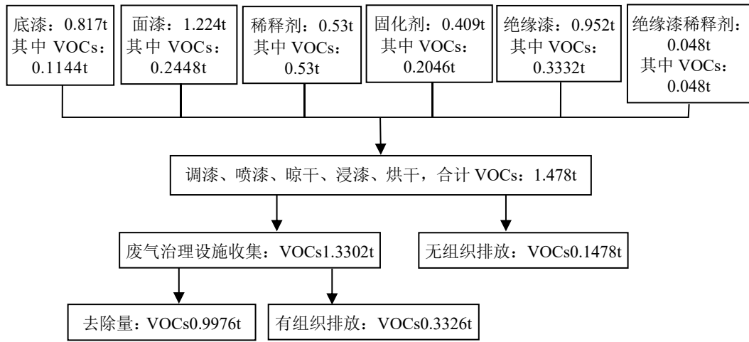
图 2-2 项目有机溶剂平衡图
